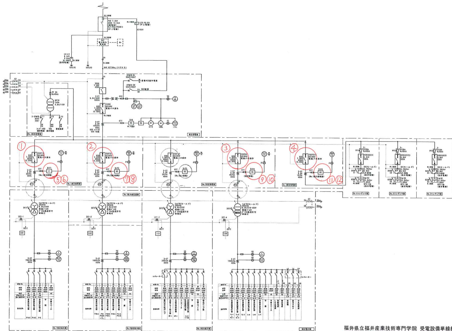
福井県立福井産業技術専門学校 受電設備単線結線図
